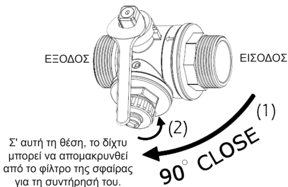
Βαλβίδα σφαίρα σε κλειστή θέση
