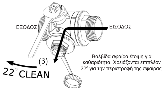
Βαλβίδα σφαίρα σε ανοιχτή θέση
